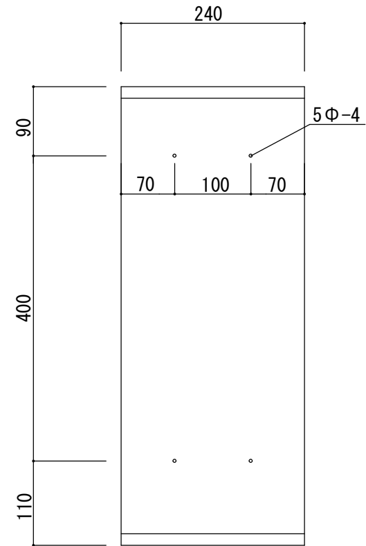
背面
